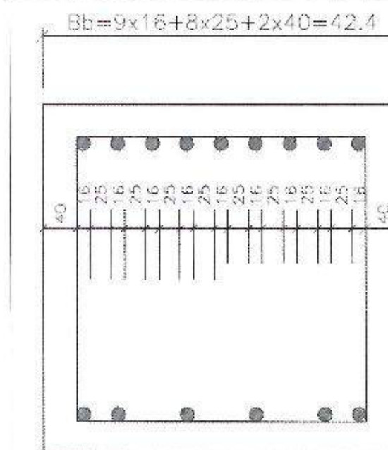
شکل ۵: مقطع عرضی تیر
