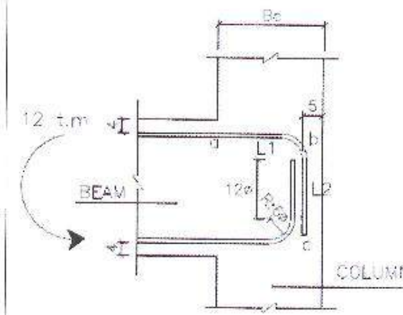
جزئیات خم کردن آرماتورهای اتصال تیر به ستون کناری
