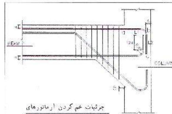
شکل ۲: کناری اتصال تیر به ستون
